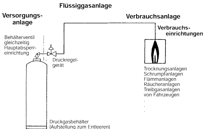
Bild 1: Flüssiggasanlage
