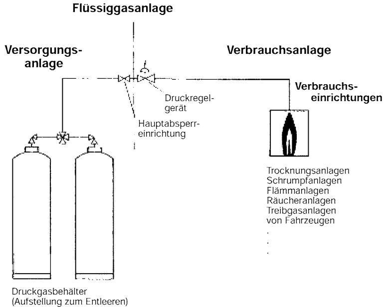
Bild 2: Flüssiggasanlage
