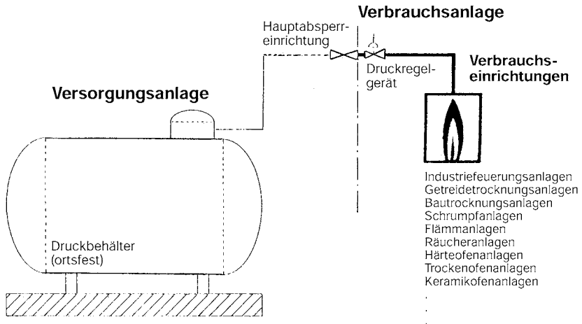
Bild 3: Verbrauchsanlage
