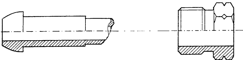
Bild 7: Pol-Anschluss von Druckregelgeräten für Druckbehälter
